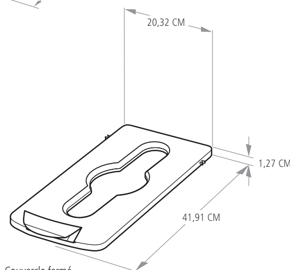
Couvercle fermé
